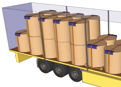
Obr. 34: Panelové blokowanie s použitím nákladnej palety
