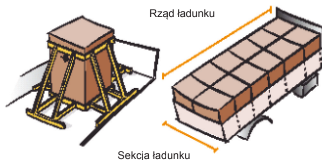
Obr. 33: Blokowanie
