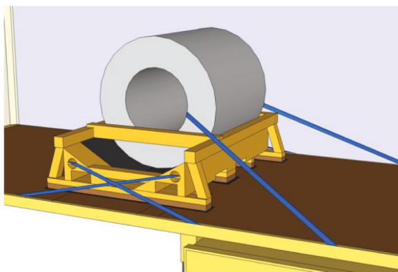
Obr. 62: Osobitná konštrukcia na prepravu zvitkov
