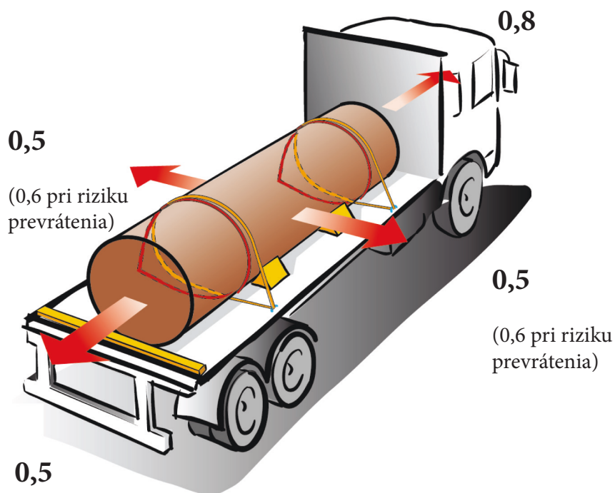
Obr. 1: Zotrvačné sily počas cestnej prepravy
