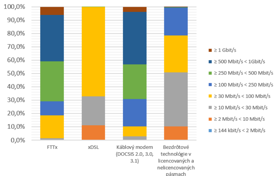
Podiel rýchlostí širokopásmových prístupov využívaných jednotlivými technológiami v roku 2025
