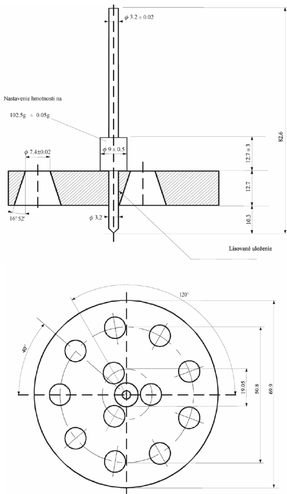
Obrázok 1 - Penetrometer
