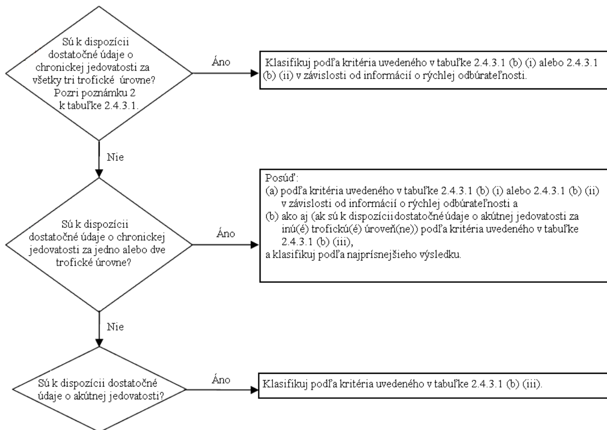
Obrázok 2.4.3.1: Kategórie látok dlhodobu nebezpečných pre vodné prostredie
