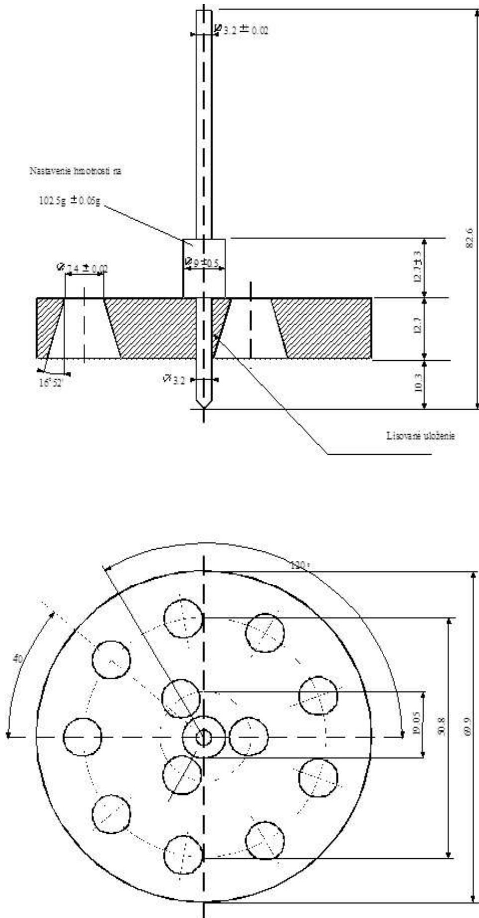
Obrázok 1 – Penetrometer
