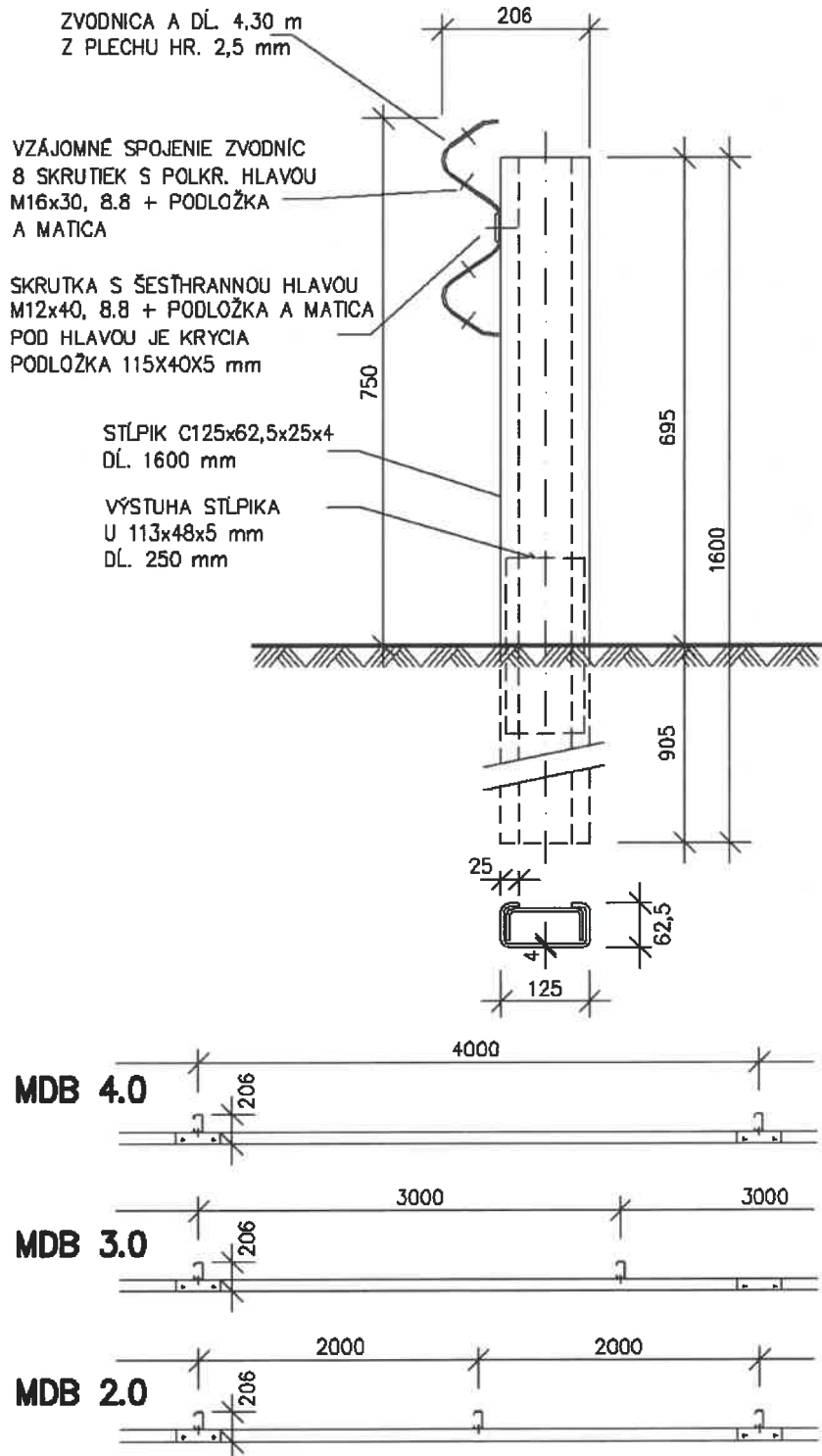
Obrázok 14 – Výrobný rad zvodidiel MDB, v [mm]
