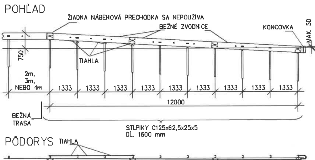
Obrázok 16 – Dlhý nábeh zvodidiel MDB, v [mm]
