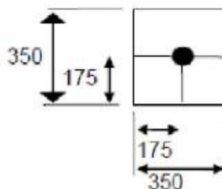
Obrázok J.1.2 – Usporiadanie s kotvou umiestnenou v stykoch vzoriek tepelnoizolačného panelu
