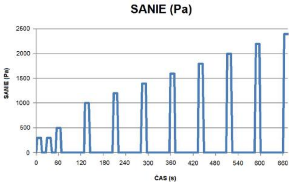
Obrázok F.2 – Príklad krokov zaťaženia vetrom
